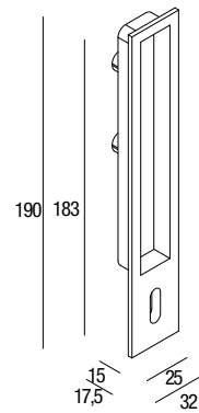
Collezione Manhattan con foro Patent "Manhattan" collection with Patent keyhole
