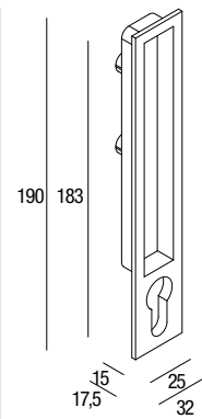
Collezione Manhattan con foro Yale "Manhattan" collection with Yale keyhole
