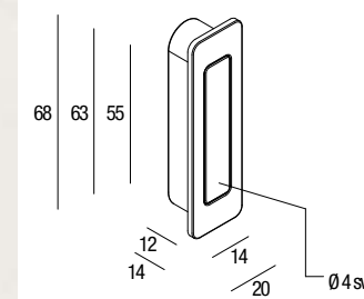
Montaggio legno, metallo Assembly on wood and metal doors
