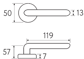
7.7 Дверная ручка на круглом основании
