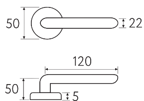
7FS Дверная ручка на круглом основании
