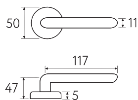
7FS Дверная ручка на круглом основании
