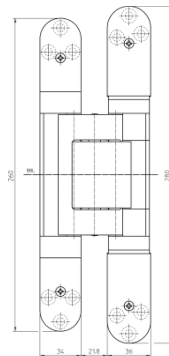
вид спереди
